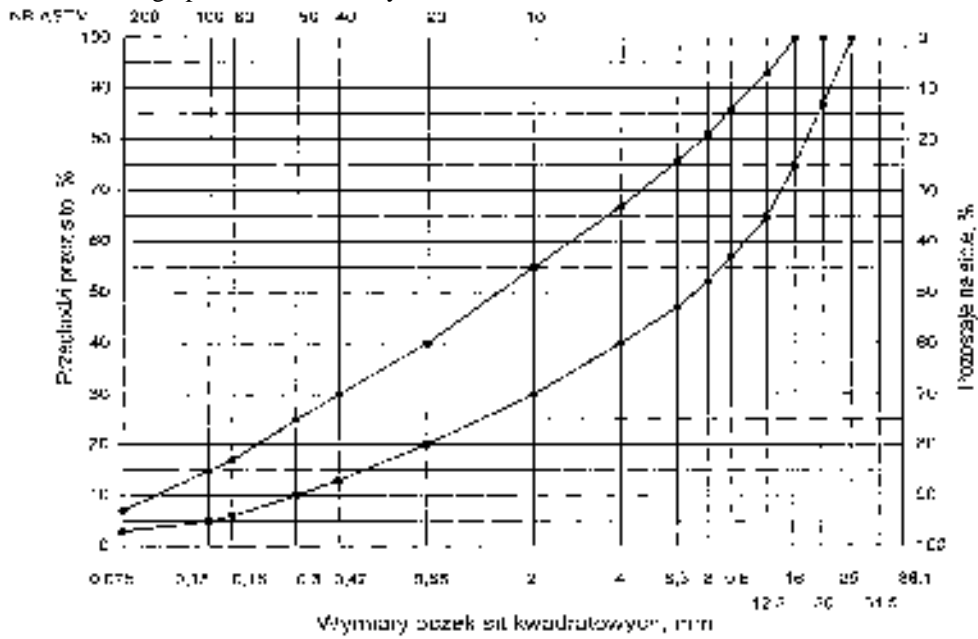
13. Rys. 8. Krzywe graniczne uziarnienia mieszanki mineralnej BA od 0 do 20 mm do warstwy wiążącej, wyrównawczej i wzmacniającej nawierzchni drogi o obciążeniu ruchem KR1 lub KR2
